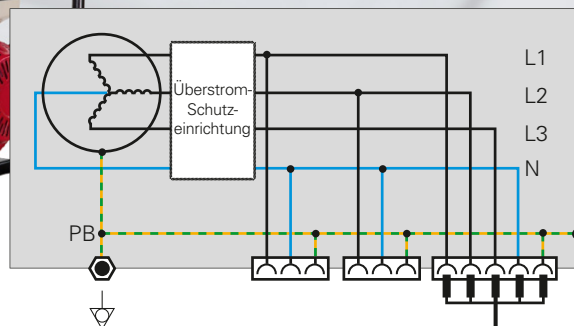
Stromerzeuger Bauart A
