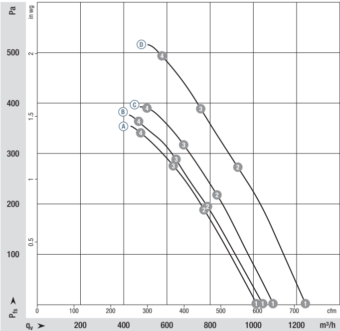
Kennlinien:
