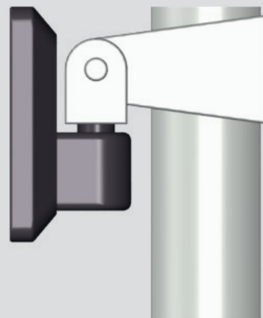
Rundrohr Ø 48 mm Anbindung von oben
