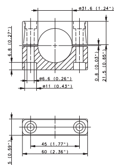
Typ BKS D32 PA Art.-Nr. 5960223002 inkl. 2 Schrauben M6 x 45 mm, DIN 912
