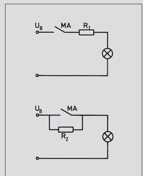
2) Lampenlast
