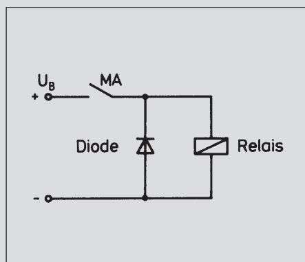
Unterdrückung von Spannungsspitzen mit einer Freilaufdiode
