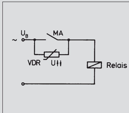
1) Spannungsspitzen beim Abschalten von induktiven Lasten werden durch Parallelschaltung eines spannungsabhängigen Widerstandes (VDR) zum Reed-Kontakt unterdrückt.
