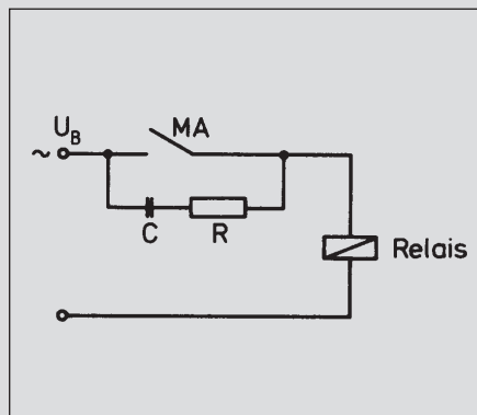
2) Ein wirkungsvoller Schutz bei Wechselfspannung ist eine Kombination aus einem Widerstand und einem Kondensator (RC-Glied).
