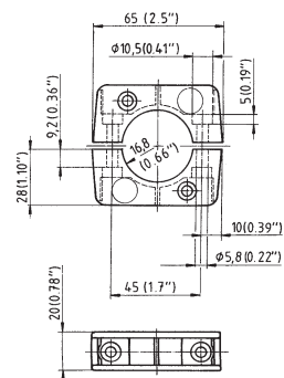
Typ BKS-D34PA Art.-Nr. 5960223041
