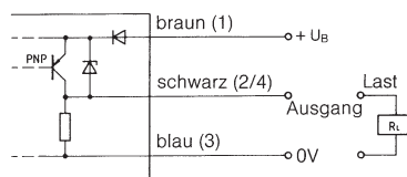
④ PNP hell schaltend oder dunkel schaltend
