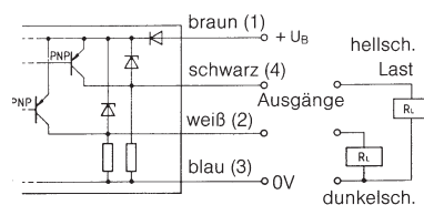
⑤ PNP antivalent hell schaltend und dunkel schaltend
