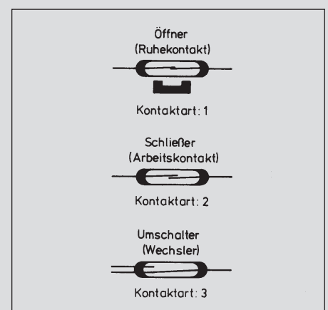
Ausführungen von Reed-Kontakten
