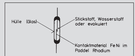
Aufbau eines Reed-Kontaktes
