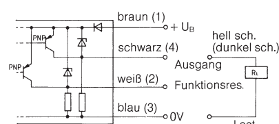
⑥ PNP hell schaltend und Funktionsreserveausgang
