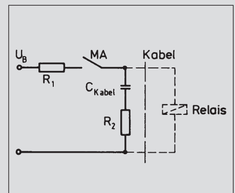
1) Kapazitive Last
