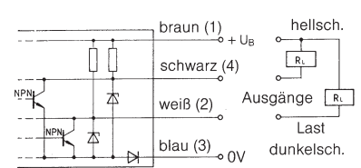
⑧ NPN antivalent hell schaltend und dunkel schaltend
