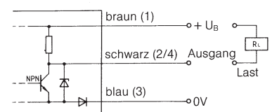
⑦ NPN hell schaltend oder dunkel schaltend
